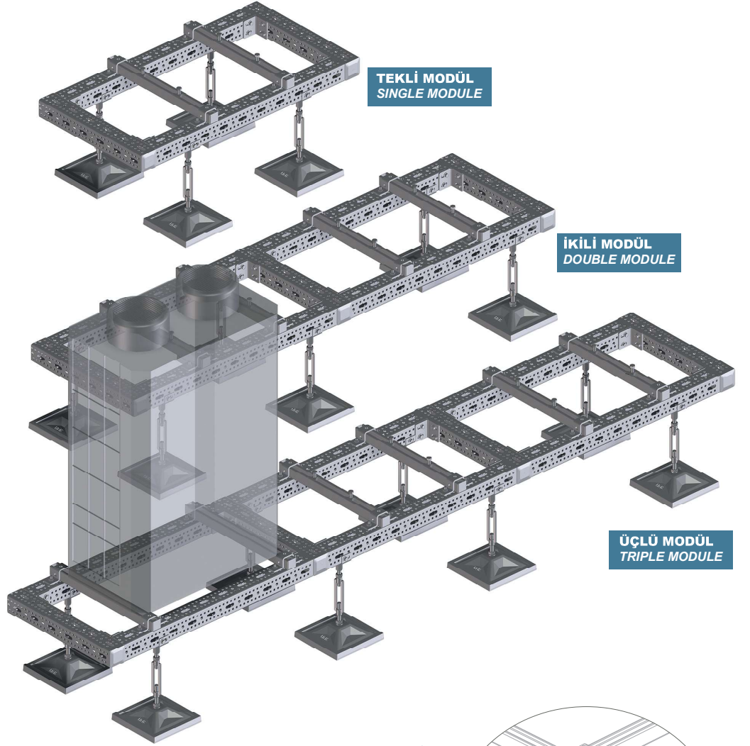
MODÜLER PROFİLLER MODULAR PROFILES
