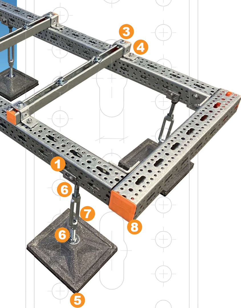
PROMEGA KÖŞE BAĞLANTI ELEMANI PROMEGA CORNER CONNECTION ELEMENT
