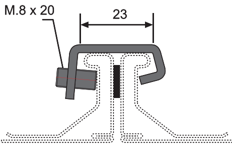
Mini Klemens • Mini Clamps LKL.350
