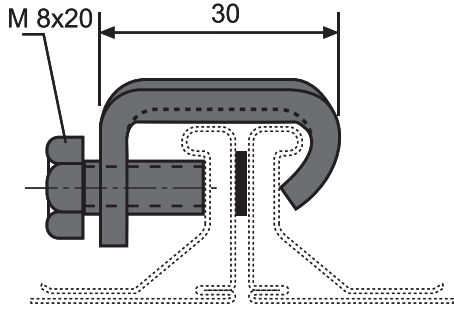
Maxi Klemens • Maxi Clamps LKL.250
